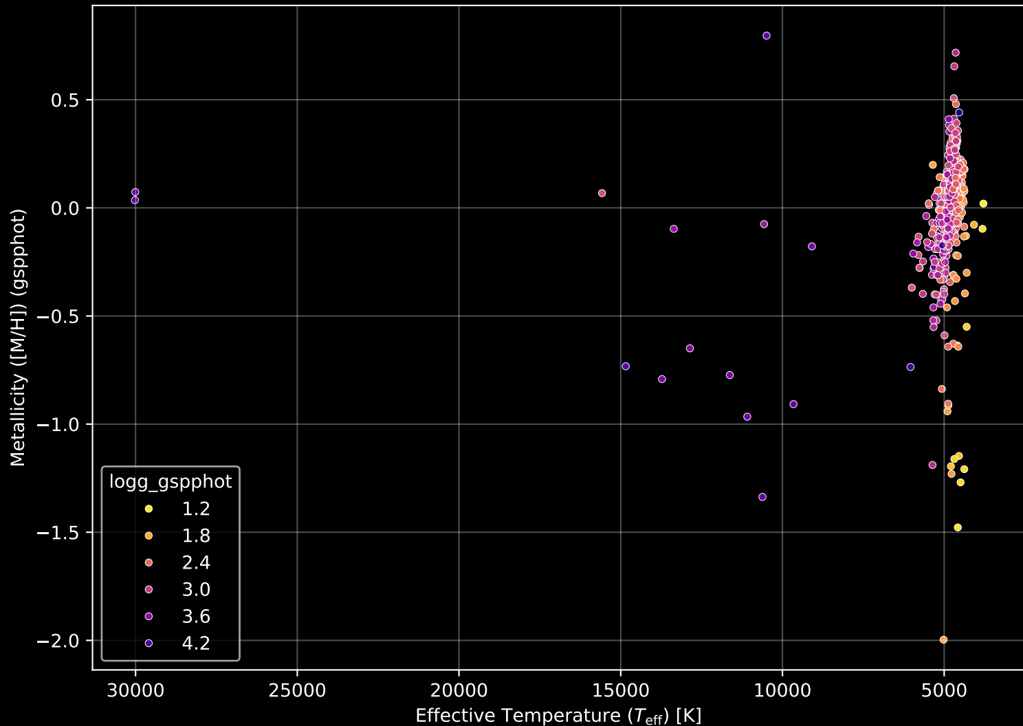
APOGEE DR17 Field: [025-06] Stellar Population Parameters (n= 561)
